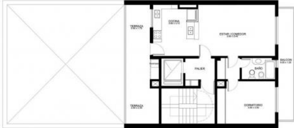
PLANTA PISO 10 ESC. 1:100
