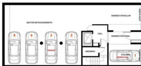
PLANTA BAJA ESC. 1:100
