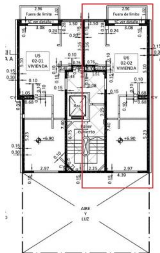
PLANTA 2º PISO Escala 1:100
